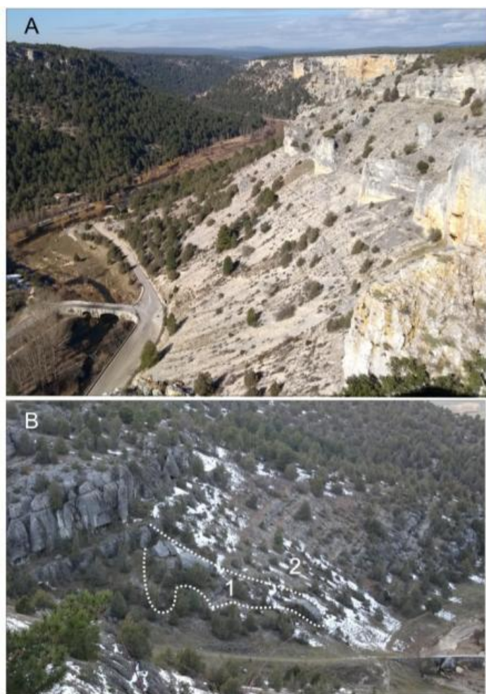
Foto 4.39. Laderas regularizadas. A, Laderas regularizadas y taludes de derrubios activos en la ladera de La Galiana, orientada al norte. B, Laderas regularizadas (1) y desprendimientos gravitacionales (2) en el flanco norte del sinclinal de Hontoria, sobre el río Lobos en el puente romano
