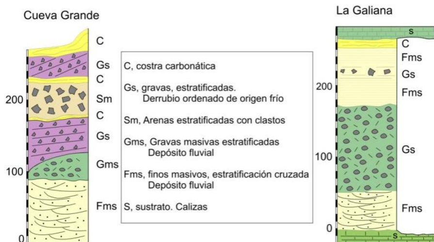
Figura 4.19. Columnas litoestratigráficas del relleno de la Cueva Grande y La Galiana Alta
