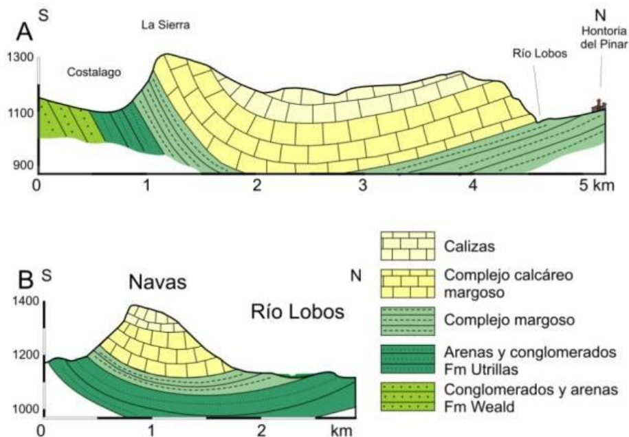
Figura 4.4. Perfiles morfoestructurales. A, Sinclinal colgado disimétrico de Hontoria. B, Sinclinal colgado de Picón. (modificado de García Fernández, 2006).
