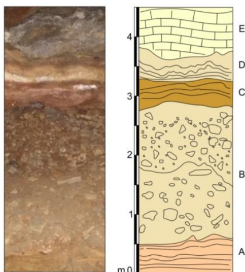
Figura 4.18. Relleno de la cueva de La Galiana Alta. A, arenas. B, derrubios de bloques y finos. C, arenas estratificadas. D, costra calcárea. E, calizas
