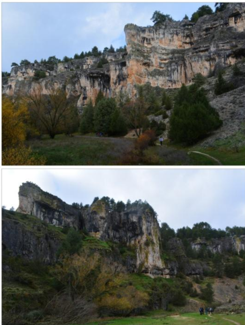
Foto 4.21. Paredes verticales del cañón del río Lobos con morfologías variadas derivadas de la incisión y abrasión fluvial y de la disolución de las calizas.
