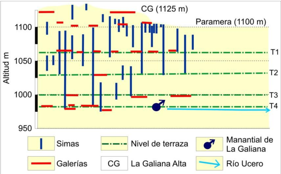
Figura 4.17. Desarrollo de las cavidades horizontales y simas en el Parque Natural, y su relación con las terrazas fluviales (Modificado de Segovia, 2008)
