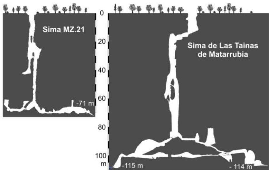
Figura 4.16. Dos ejemplos de cavidades de desarrollo vertical y perfil en T invertida ( \perp ). (Fuente: GET, 1997).
