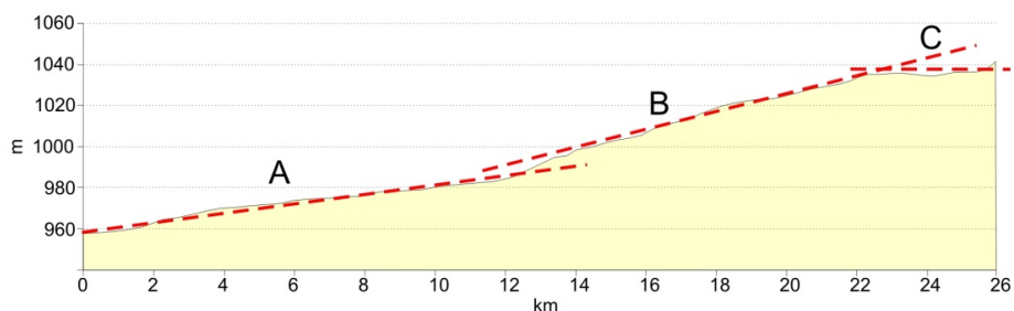
Figura 4.10. Perfiles del río Lobos en el interior del Parque Natural
