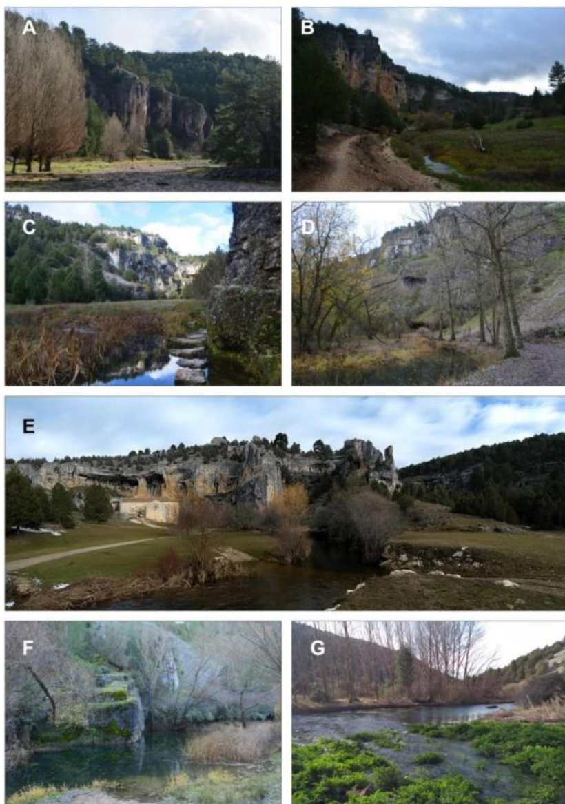
Foto 4.36. El cauce del río Lobos, el Puente de los Siete Ojos y Ucero. A, cauce seco formado por sedimentos del nivel de acumulación fluvial en Pieza Bajera. B, caudal bajo de invierno sobre formaciones fluviales de fondo de valle. C, relleno fluvial y turboso en zonas encharcadas y exutorios del sector de Las Fuentes. D, meandros sobre sedimentos fluviales en la porción media. E, caudal canalizado aguas abajo de San Bartolomé. F, cauce y exutorios en Valdecea. G, confluencia del Lobos con el Nacedero del Ucero.
