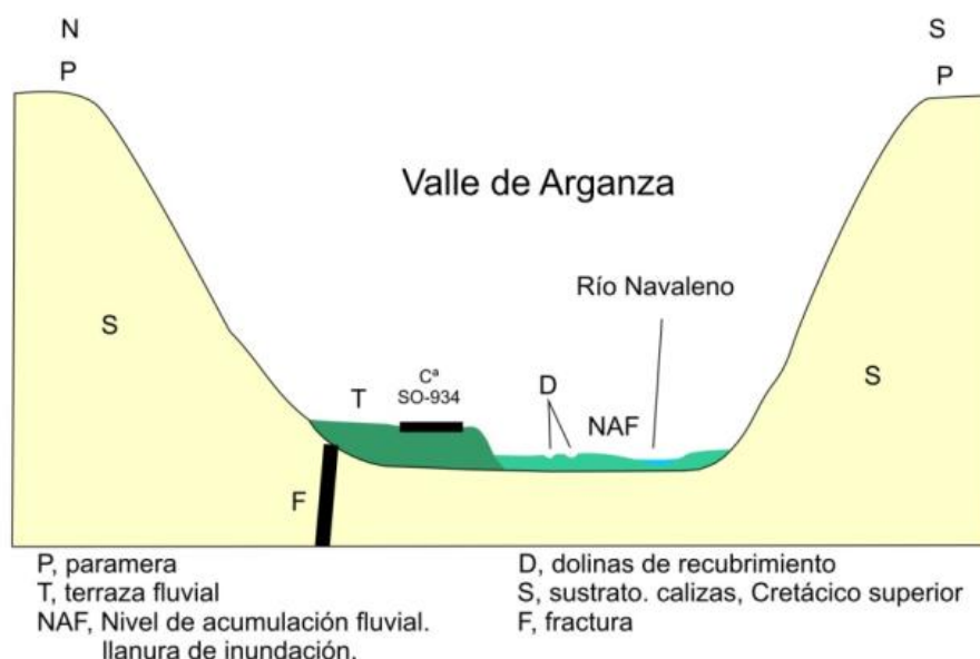
Figura 4.22. Esquema morfológico del valle del Arganza. Valle en línea de falla modelado por la acción fluvial que genera la terraza y con importantes procesos kársticos, como las dolinas de recubrimiento de la llanura de inundación
