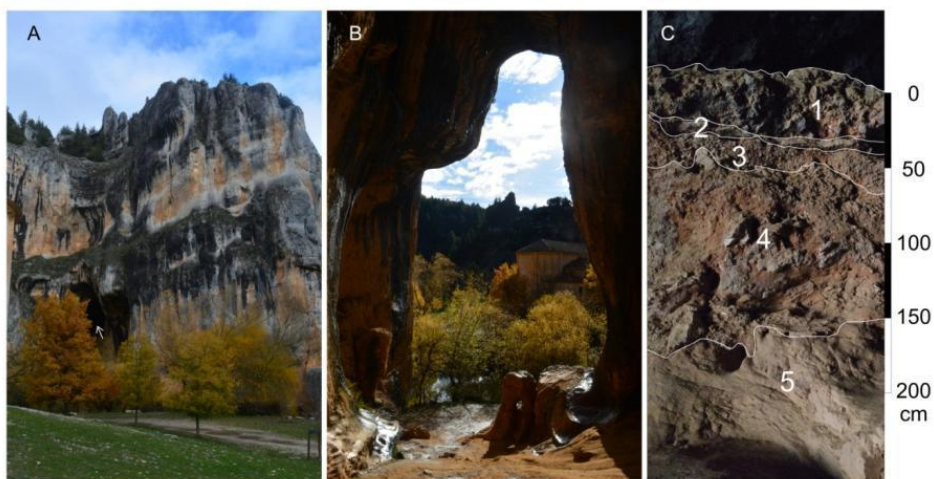
Foto 4.29. Cueva Grande. A, La flecha indica la localización de la entrada. B, Vista desde el interior. C, Relleno clástico. 1, depósito de caídas y desprendimientos. 2, costra calcárea. 3, derrubios ordenados, clastos homométricos. 4, depósito de caídas y desprendimientos, 5, sustrato arenoso.
