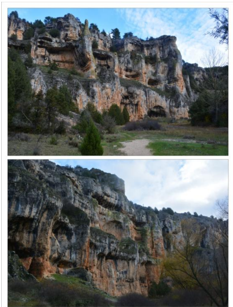
Foto 4.18. Paredes del cañón del río Lobos. Configuran el valle encajado entre las paredes calcáreas donde alternan los modelados kársticos (cavidades, bóvedas, balmas o espeleotemas), con desprendimientos y caídas dirigidos por la estratificación y el diaclasado.
