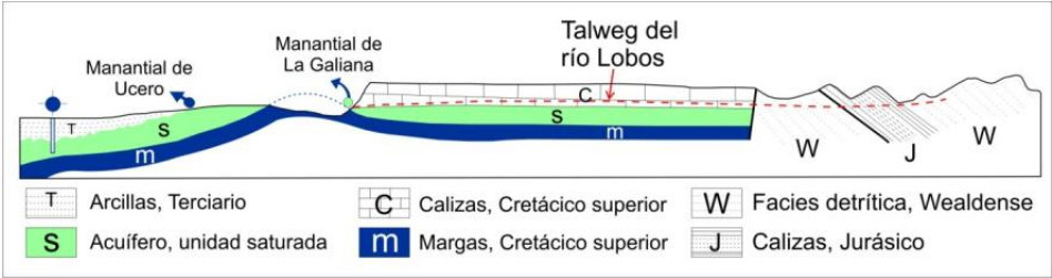
Figura 4.14. Esquema hidrogeológico N-S del acuífero del Cañón del Río Lobos (Modificado de Segovia, 2008)
