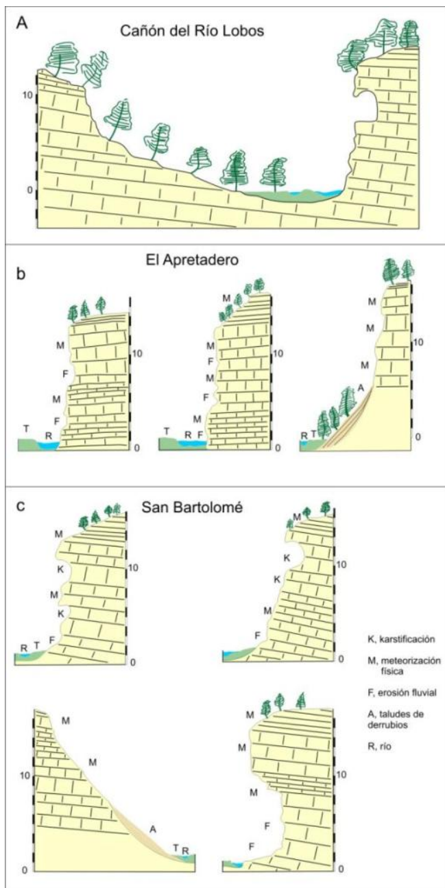
Figura 4.7. Laderas del Cañón del río Lobos. A, disimetría característica de la morfología del cañón. B, morfología de las paredes en el sector de El Apretadero. Dominio de la meteorización física y la erosión fluvial. C, morfología de las paredes del sector de San Bartolomé. Procesos kársticos, fluviales y meteorización en las paredes.
