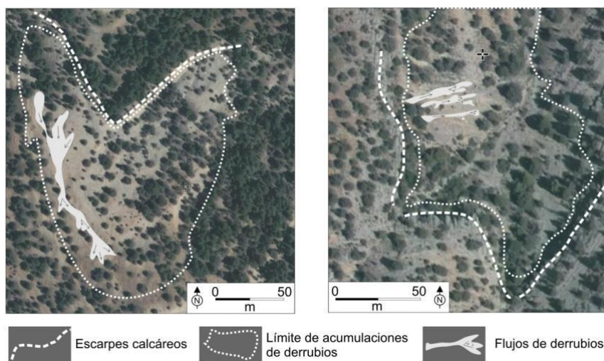
Figura 4.26. Acumulaciones de derrubios heredados y parcialmente activos con flujos de derrubios en la Sierra de Nafría (A) y en la Sierra de Hontoria (B)
