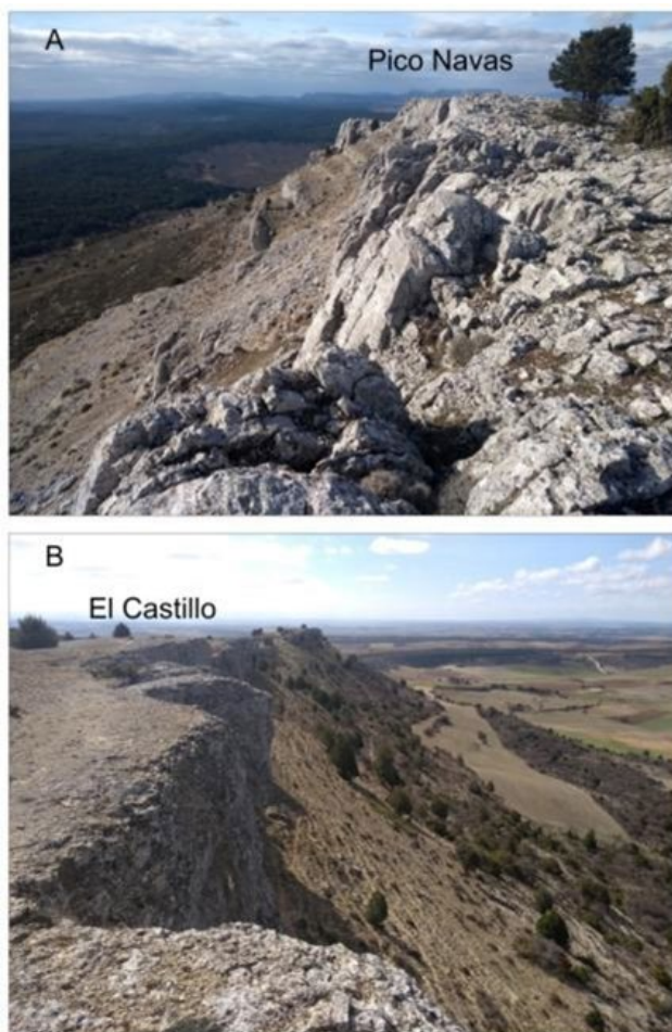
Foto 4.40. Sistemas de cantil talud en las laderas del Parque. A, Cantil escalonado en las calizas y talud de derrubios en las laderas del sinclinal colgado de Navas. B, Cantil y laderas regularizadas en El Castillo.
