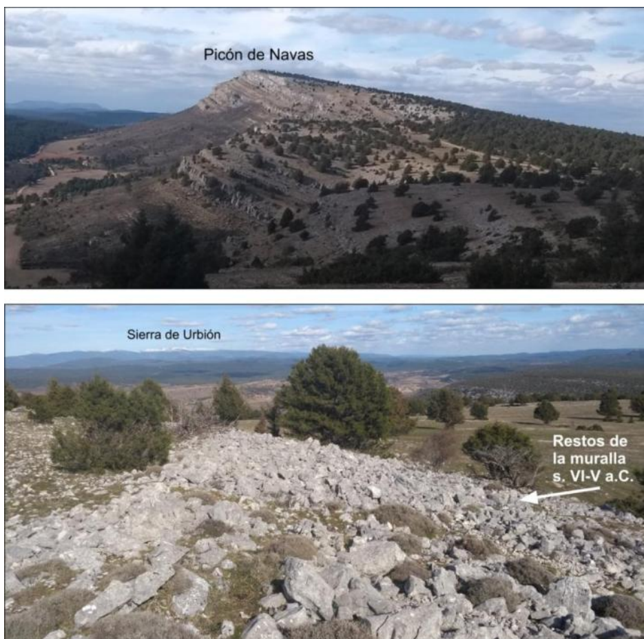
Foto 6.5. Porción del LIGm nº6. Sinclinal colgado del Picón de Navas. Arriba, vista general del flanco sur desde el oeste. Abajo, amplio paisaje sobre las parameras y montañas sorianas, al fondo, y restos de la muralla del castro que ocupó la cumbre en primer plano.
