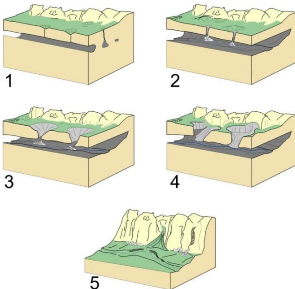
Figura 4.8. Modelo de evolución holokárstica y génesis de un cañón.
