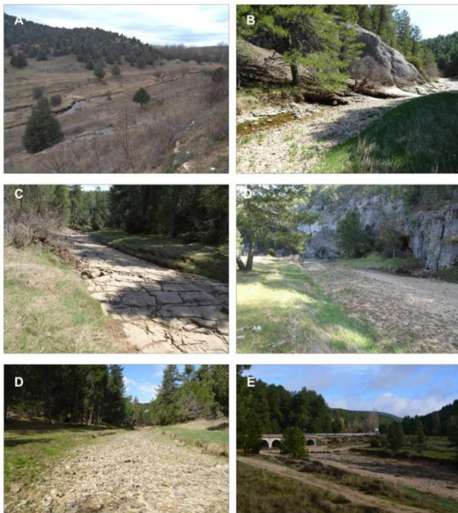
Foto 4.35. El cauce del río Lobos entre Hontoria y el Puente de los Siete Ojos. A, sobre sedimentos del nivel de acumulación fluvial en las proximidades del puente medieval. B, cauce seco formado por cantos y bloques fluviales en las proximidades de Las Raideras. C, talweg sobre el sustrato calcáreo. D, meandros y cauces rectilíneos sobre sedimentos fluviales. E, llanura de inundación en el Puente de los Siete Ojos.
