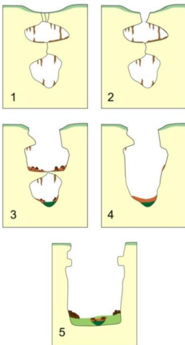
Figura 4.9. Evolución holokarstica en el cañón del río Lobos.
