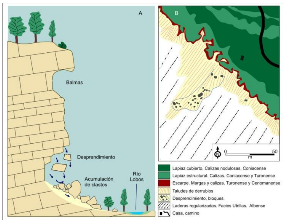
Figura 4.23. Desprendimientos en el escarpe de La Sierra, en la ladera septentrional de Costalago
