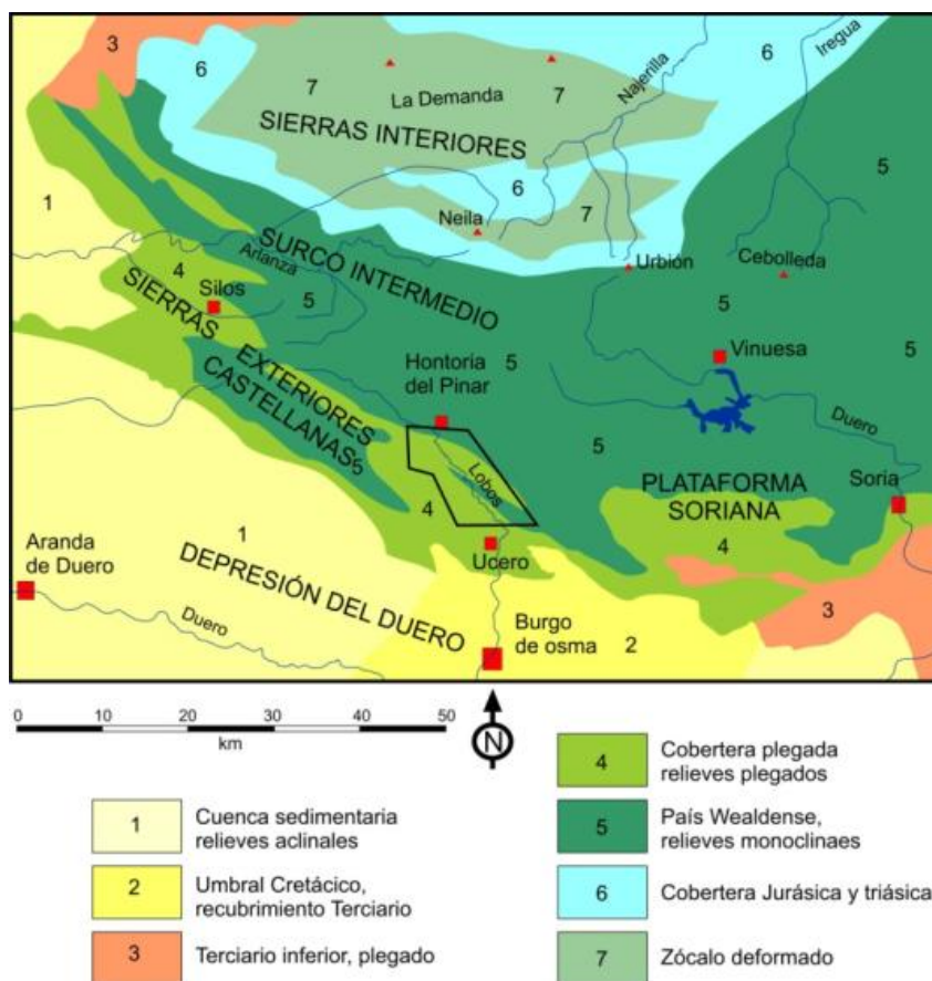
Fig 4.1. Esquema estructural del contexto de la zona de estudio. Cuadro negro, Parque Natural del Cañón del Río Lobos.
