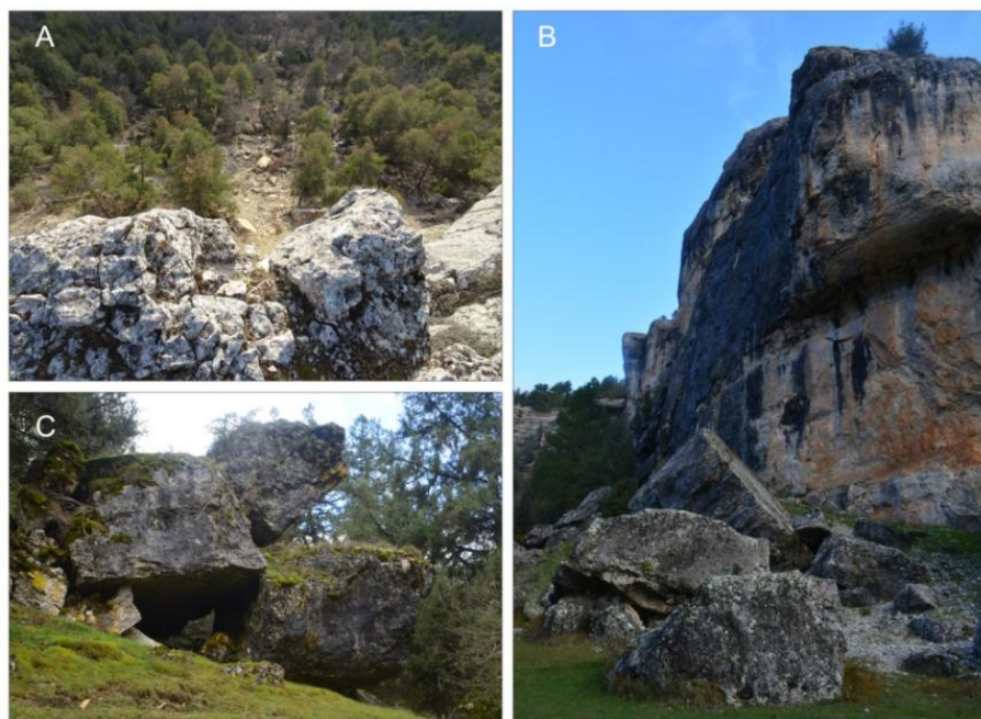
Foto 4.37. Desprendimientos en las laderas del Parque. A, Desprendimientos y acumulaciones de clastos en la Sierra de Hontoria. B, Desprendimientos en las paredes del río Lobos. C, Acumulación de bloques por desprendimientos gravitacionales en el cauce del río Lobos.
