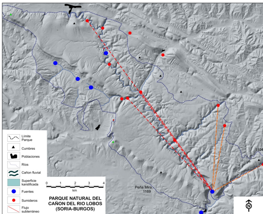
Figura 4.15. Flujos de drenaje desde las zonas de infiltración hacia las fuentes (Fuente, Segovia, 2008)
