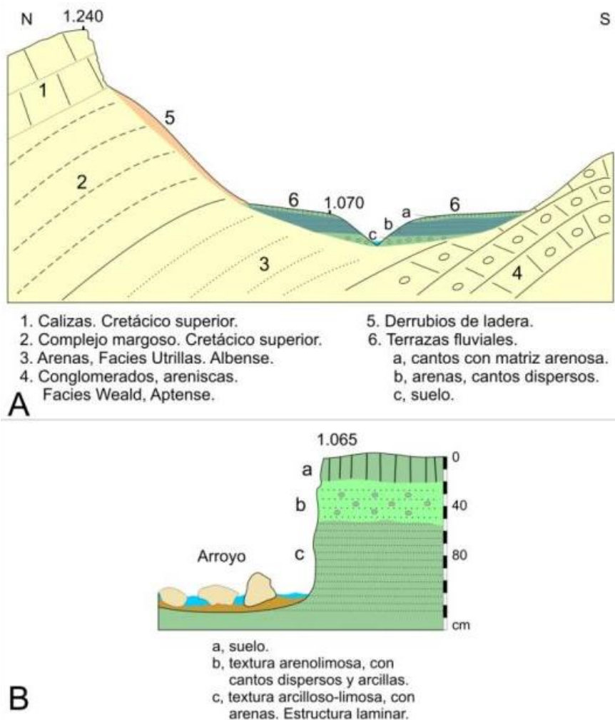
Figura 4.21. Costalago. A, esquema morfológico. B, columna del relleno lacustre de la parte central del valle de Costalago
