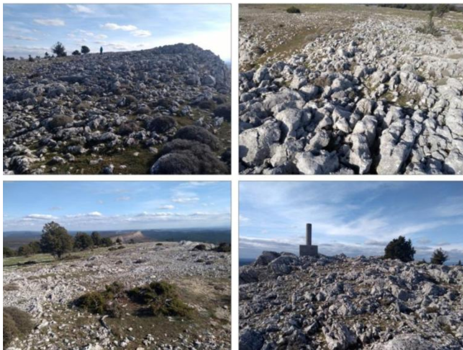
Foto 4.22. Lapiaces en el Picón del Navas. Lapiaces estructurales elaborados en la culminación del sinclinal colgado de Navas, sobre las calizas de la Formación Hontoria del Pinar (Santoniense inferior).
