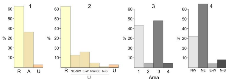
Figura 4.11. Porcentaje de dolinas por tipo. 1. Distribución por tipo. R, redondeadas. A, elípticas. U, uvalas. 2. Porcentaje por tipo y alineación. 3. Porcentaje de representatividad por unidad kárstica. 4. Porcentaje por orientaciones.
